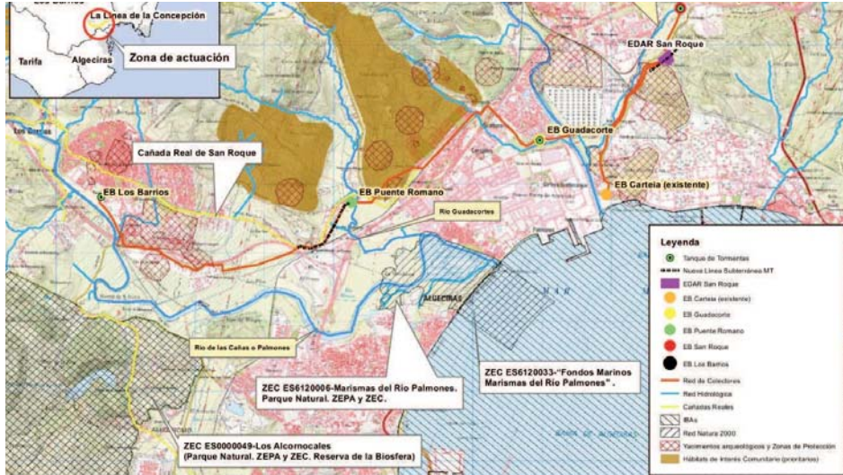
Plano de las actuaciones, con la nueva EDAR de San Roque y la agrupación de vertidos de los distintos núcleos sanroqueños y de Los Barrios. VCG
