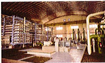
Estación desaladora de Fonsalla, en Guía de Isora. ANDRÉS GUTIÉRREZ
